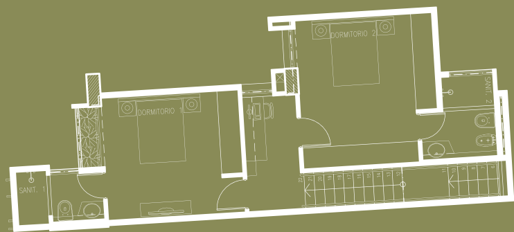
NIVEL SUPERIOR (+3,50)
