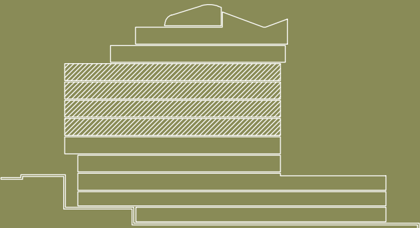
UBICACION DE LAS 8 UNIDADES EN CORTE LONGITUDINAL (NIVELES +7,00; +11,50; +14,00 Y 17,50)
